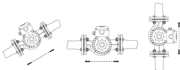
Рис. 57 Варианты монтажа
